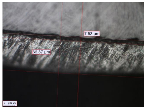
Bild: Schichtaufbau, Stahl-Hartzink-Zinklegierung
