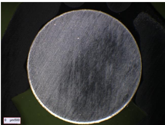
Bild: Querschliff eines beschichteten Drahtes
